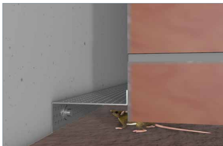
▲ Ungezieferschutz: Lochblech
