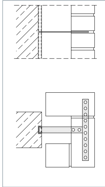
▲ Zur Pfeilverankerung
