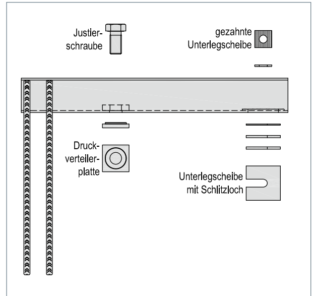
▲ Attikausführung FB-EJA
