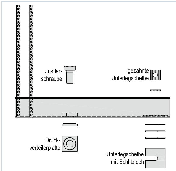
▲ Standardausführung FB-EJ
