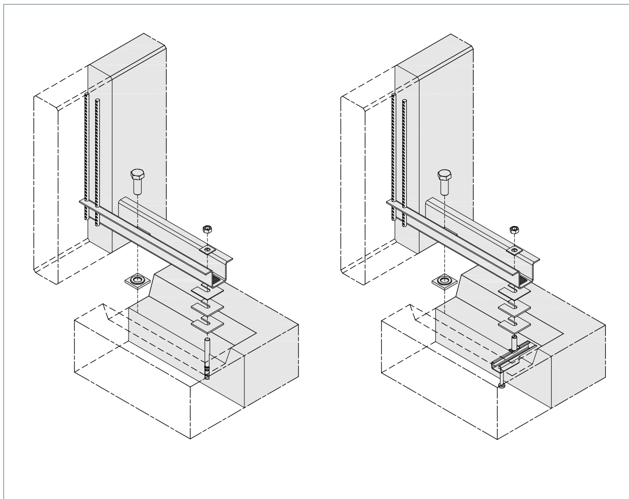
▲ FB-EJ: Dübelbefestigung
