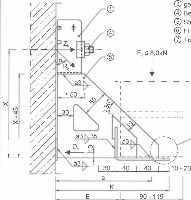
Seitenansicht
