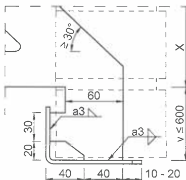
Versatzkonsole
