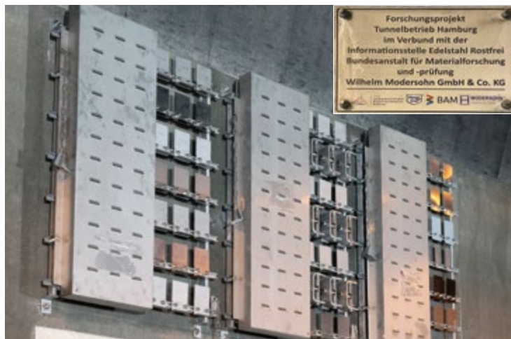
▲ Montage der Werkstoffproben im Elbtunnel Hamburg, im Rahmen eines Forschungsprojektes zur Erweiterung des Anwendungsbereiches des Werkstoffes 1.4462.
