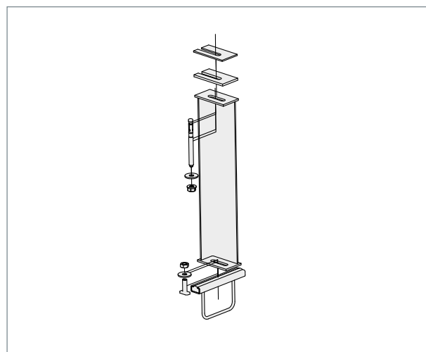
▲ Explosionszeichnung FB-I
