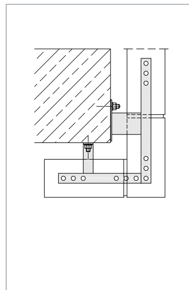
▲ Für L-förmige Sturzausbildung
