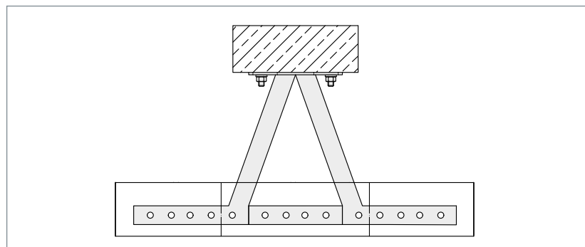
▲ Horizontale Sicherung eines langen Mauerwerks Pfeilers mit schmaler Stahlbeton-Stütze im Rohbau als Verankerungsgrund
