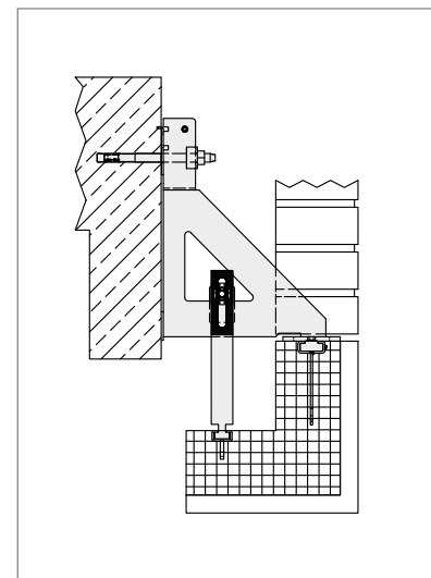
▲ Fertigteil mit Kippsicherung (ZK-Lasche) an Standard FB-U Konsole
