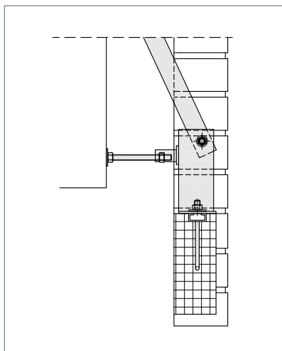
▲ Eckkonsole für Fertigteile FB-ZBV
