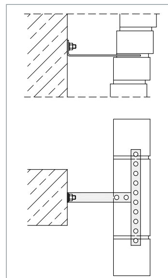
▲ Für abgetrepptes Mauerwerk
