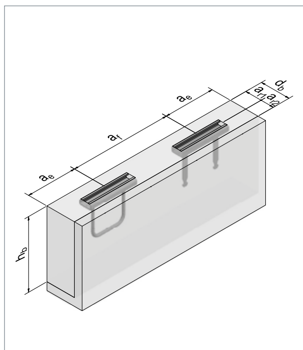
▲ Links MBA 38/18 ES, rechts MBA 38/17 ESF
