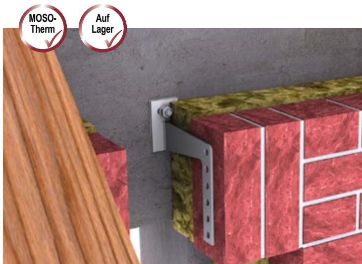
▲ Sturzabfangung mit MOSO® Einzelkonsolanker EK-G
