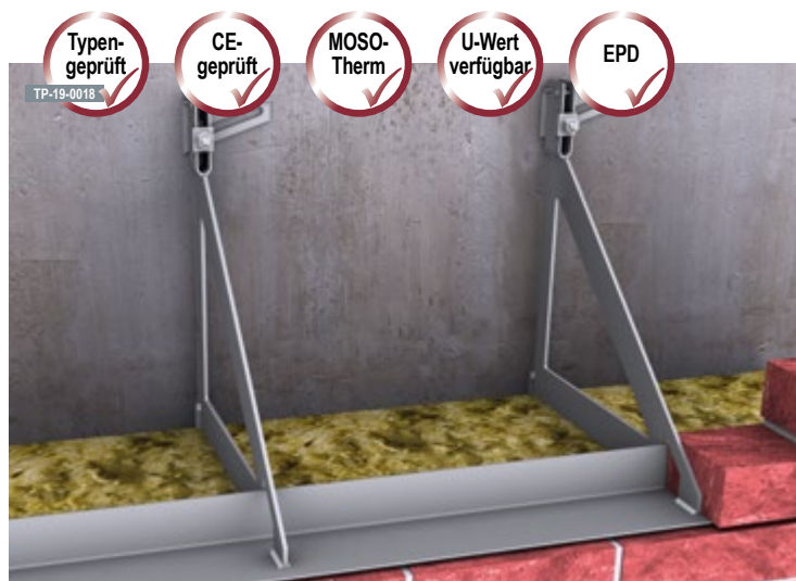
▲ Wandabfangung mit MOSO® Winkelkonsolanker WK-N
