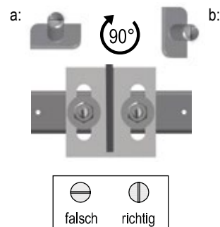
Detailansicht MHK-Schraube im Einbauszustand
