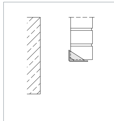
▲ WA-Ü mit Aussteifungsblech
