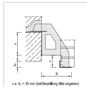
▲ WK-OV mit Versatz
