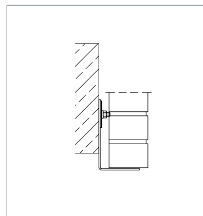
▲ Mit Höhenjustierung
