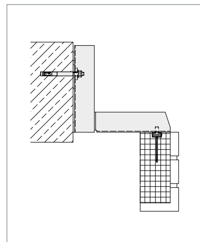
▲ FB-G, Höhenlage unten
