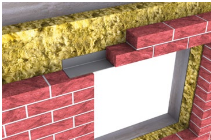
▲ Öffnungsüberdeckung mit MOSO® Winkelaufleger WA-Ü
