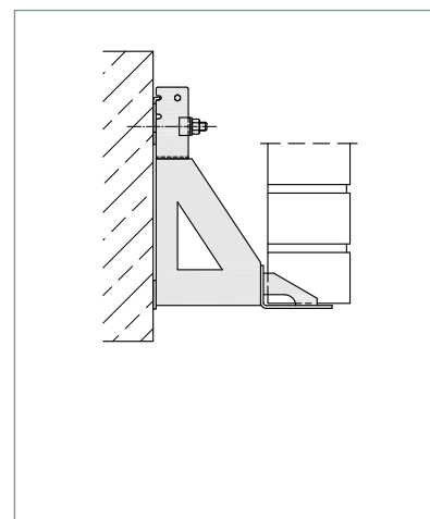
▲ WK-NX mit eingeschweißtem Knotenblech
