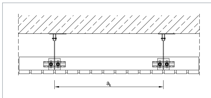
▲ Fertigteilbefestigung FB-U
