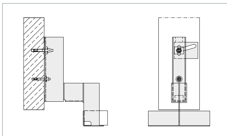
▲ Einzelanker Montage am schmalen Rohbau, 2. Dübel als Verdrehsicherung
