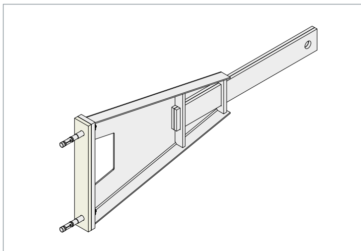
▲ Sonderdauergerüstanker für große Schalenabstände
