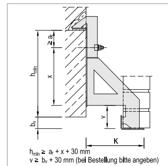
▲ WK-KV mit Versatz
