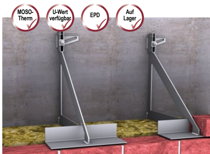
▲ Wandabfangung mit dem MOSO® Einzelkonsolanker EK-L
