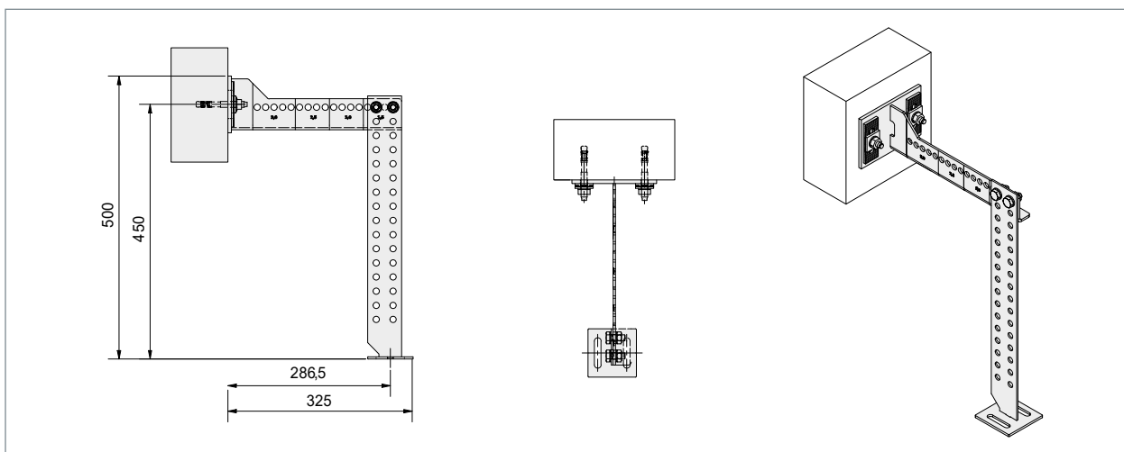
▲ Die Bauform der FB-R erlaubt Verankerungen z.B. an Stahlbeton-Decken
