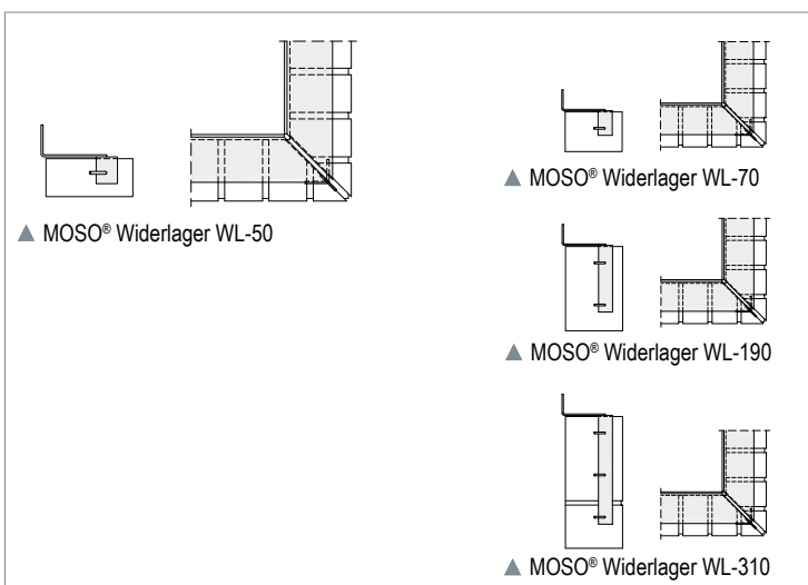
▲ Diverse Widerlager im Eckbereich, Typ WL
