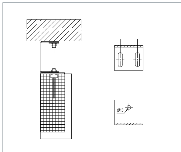
▲ FB-IS Sonderbauform für schmale Abstände
