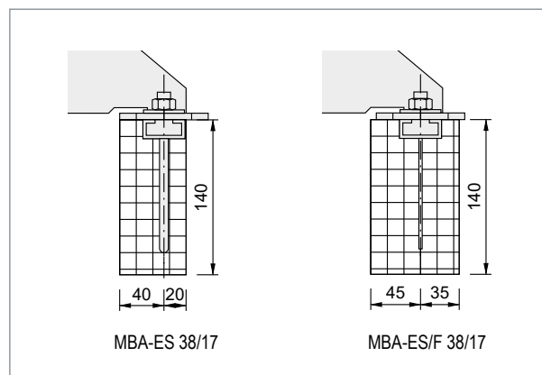
▲ MOSO® MBA-ES und MBA-ESF 38/17
