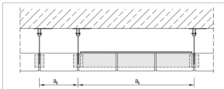
▲ Mit dem Zwischenwinkel WA-Z lassen sich verschiedene Ankerabstände einstellen
