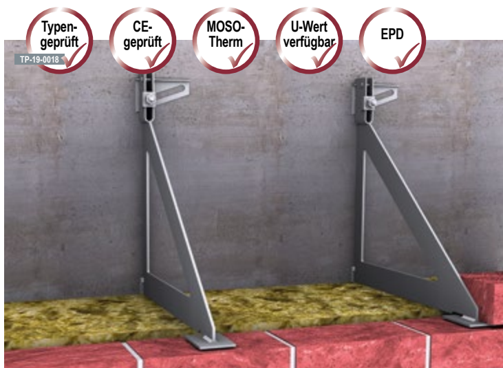
▲ Wandabfangung mit dem MOSO® Einzelkonsolanker EK-U
