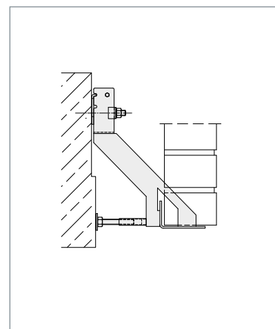
▲ Druckschraube \pm 15 mm justierbar
