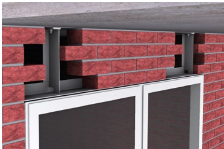
▲ WK-I Konsole unter Balkonplatte
