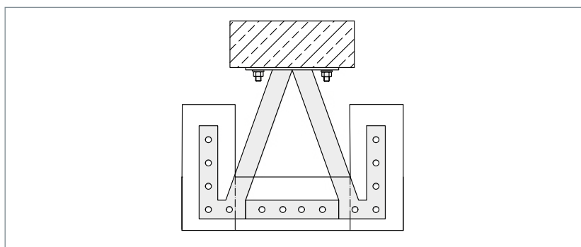
▲ Horizontale Sicherung eines U-förmigen Mauerwerks Pfeilers
