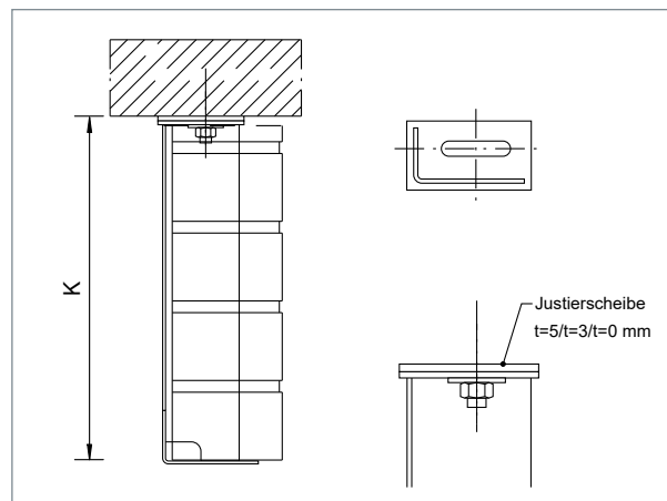
▲ WK-I Konsole
