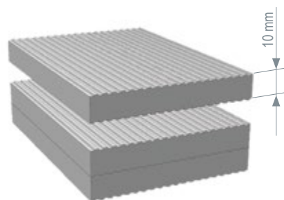
▲ Profilierte, gestapelte Dämmplatten Verfügbar in Plattenstärken von 5 mm und 10 mm
