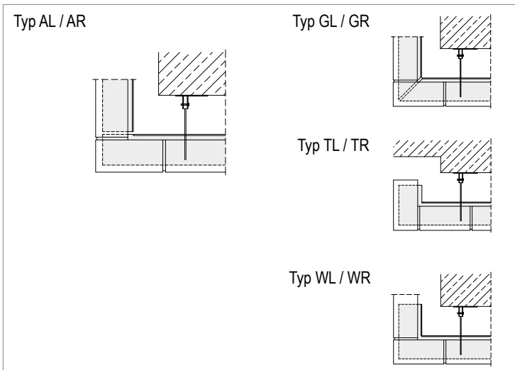
▲ Diverse Eck- und Randausbildungen
