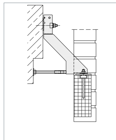
▲ FB-D mit langer Druckschraube
