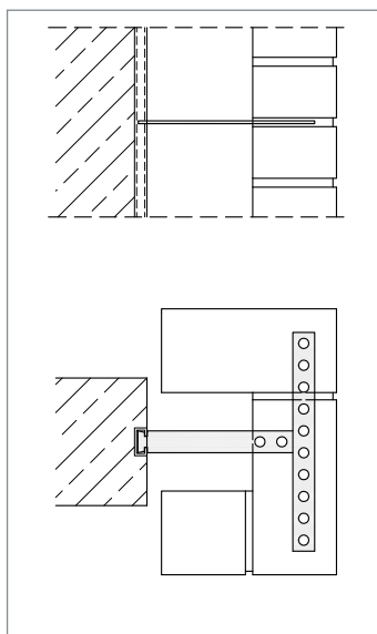
▲ Zur Pfeilverankerung
