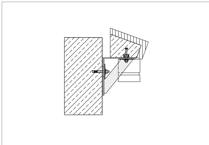
▲ Fensterbankhalter freitragend mit Verschraubungen in CE-Schiene
