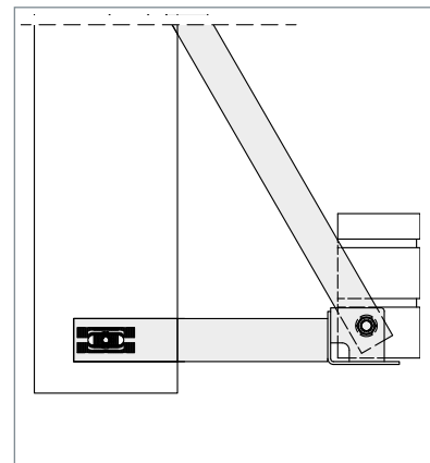
▲ WK-ZS mit Flachabstützung in Flucht der Stahlbeton-Rohbaukante
