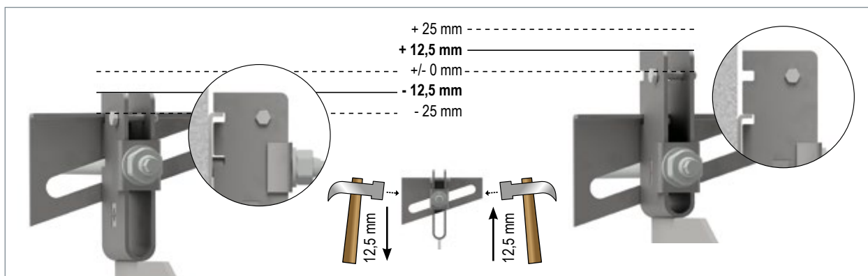
▲ ... Traganker durch Umsetzen der gekrüpfen Keilscheibe in der Höhe grob und durch Verschieben der Keilscheibe fein justieren...
