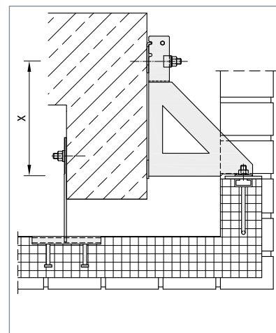
▲ FB-U mit FB-ZK als Halterung der Fertigteildecke
