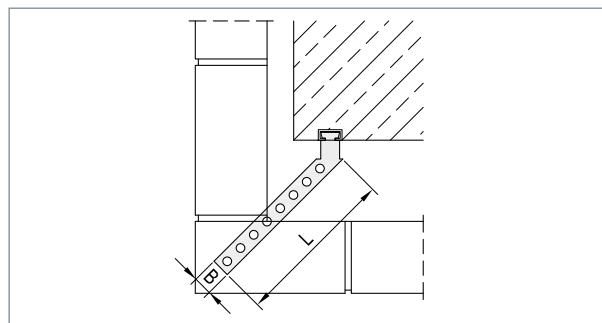
▲ MOSO® Maueranker MA-AW
