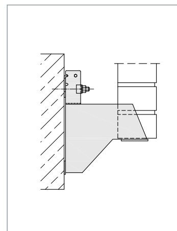
▲ Mit hochgestellter Auflagerplatte
