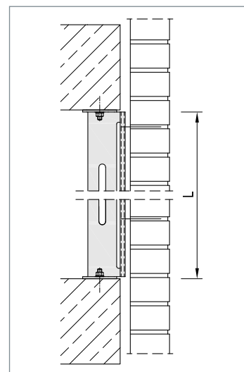
▲ Windpostanker HV-WPS zwischen Stahlbetondecken
