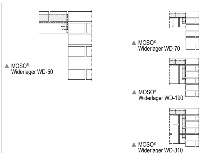
▲ Diverse Widerlager im Dehnfugenbereich, Typ WD
