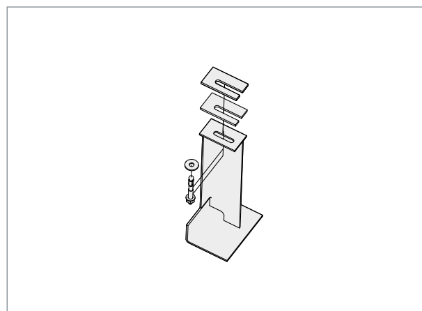
▲ Explosionszeichnung WK-I
