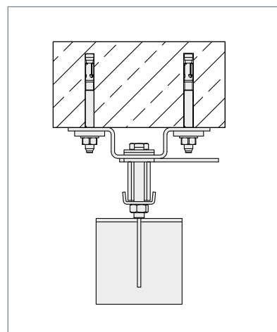
▲ Ab 20 mm: Hutprofil zwischen Rohbau und Konsole
