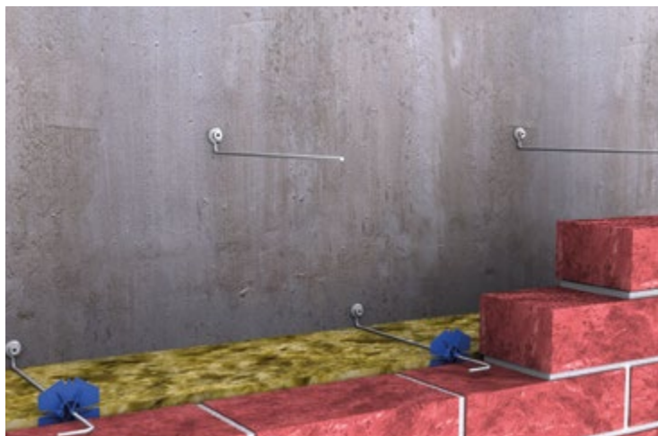
▲ Verankerung mit MOSO® Horizontalverbindung HV-L
