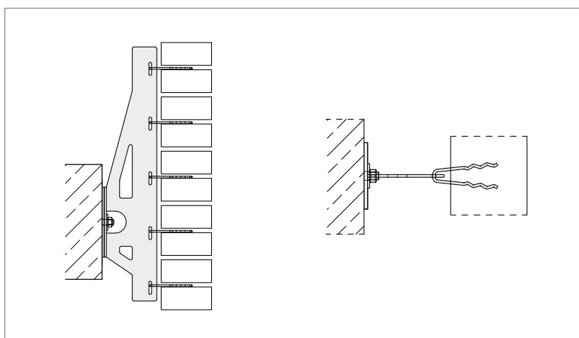
▲ HV-AS Lösung ohne MOS Schiene
