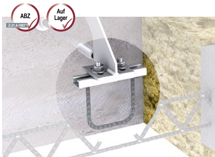
▲ Fertigsturz mit einbetonierter MOSO® Ankerschiene MBA-ES
