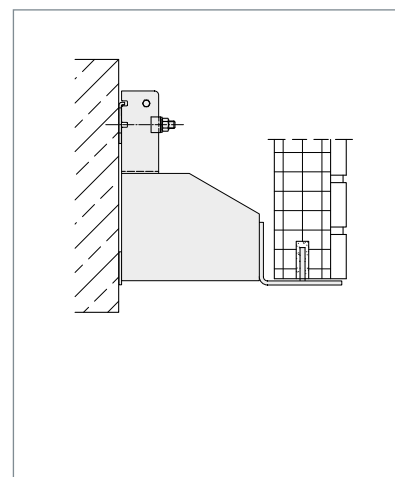
▲ EK-WS mit Dorn
