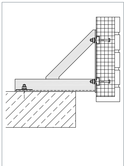
▲ Für Verankerung von Gesimsbändern
