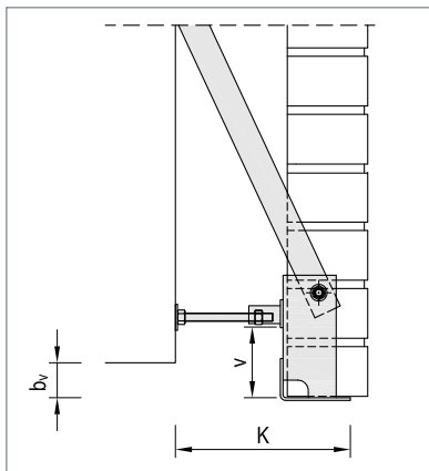
▲ WK-ZV mit Versatz
