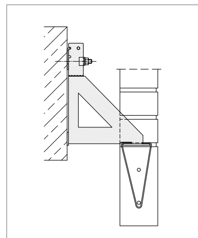
▲ EK-U mit Drahtbügel Typ 2
