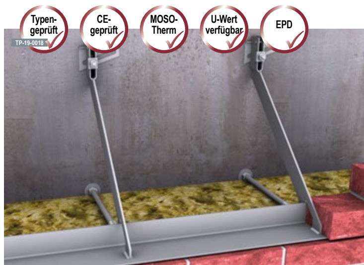
▲ Wandabfangung mit MOSO® Winkelkonsolanker WK-D
