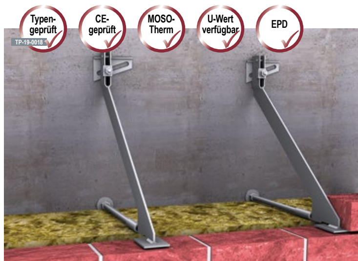
▲ Wandabfangung mit dem MOSO® Einzelkonsolanker EK-D
