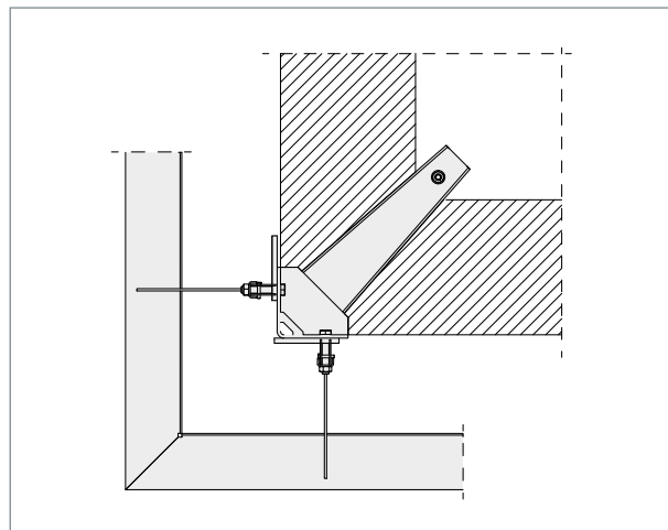
▲ Eck-Variante
