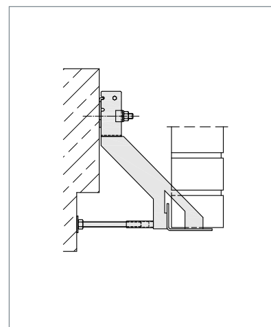
▲ WK-DS mit längerer Druckschraube
