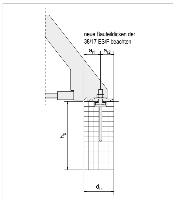
▲ Mindest-Betonkernabmessungen, gemäß Zulassung
