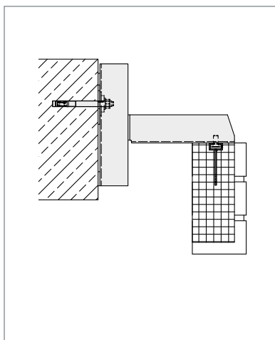
▲ FB-G, Höhenlage mittig
