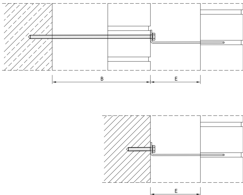
▲ MOSO® Horizontalverbindung HV-L, Verankerung in Lochstein möglich
