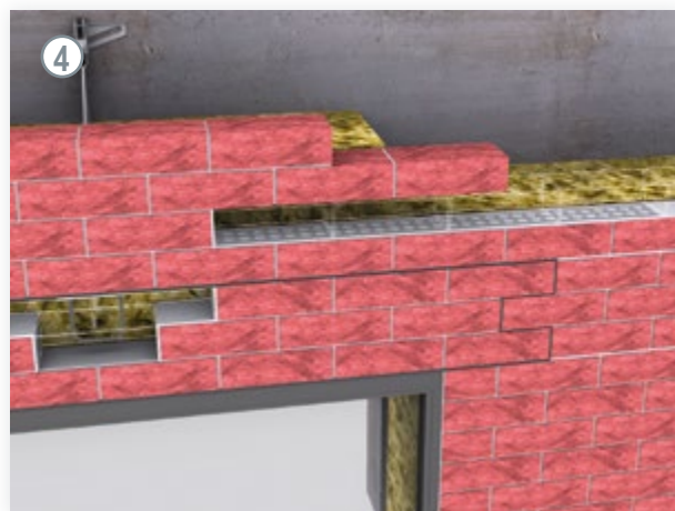
▲ Einseitig aufgelegter Fertigteilsturz
