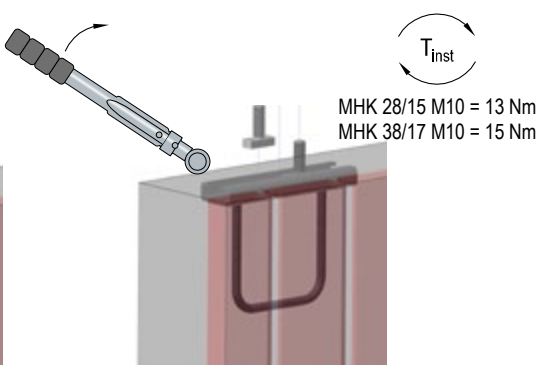
Detailansicht MHK-Schraube im Einbauszustand
