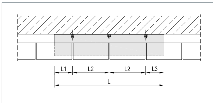
▲ Winkelaufleger WA-M als Fußpunktabfangung
