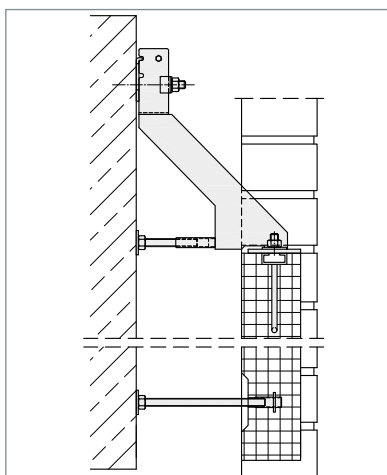
▲ FB-D mit zusätzlicher Druckschraube
