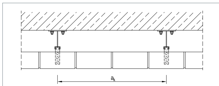
▲ Windpostanker mit variablen Abständen a_k
