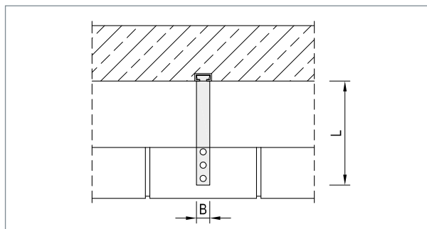
▲ MOSO® Maueranker MA-A
