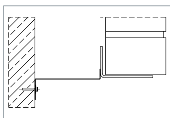
▲ Lochblechprofil
