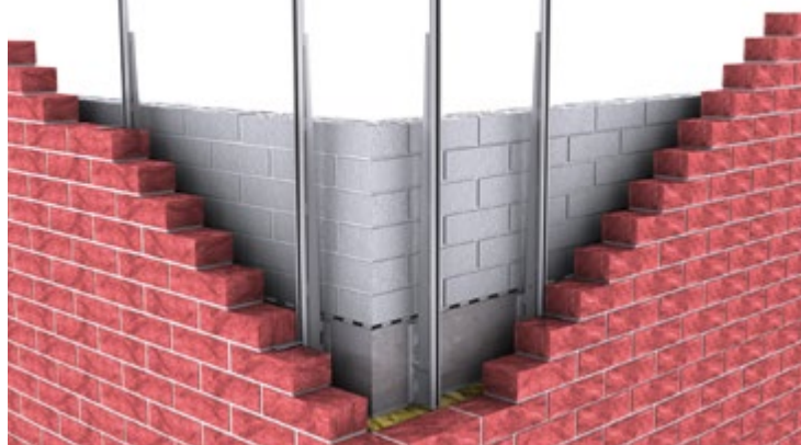
▲ Attikaverankerung mit MOSO® Horizontalverbindung HV-A
