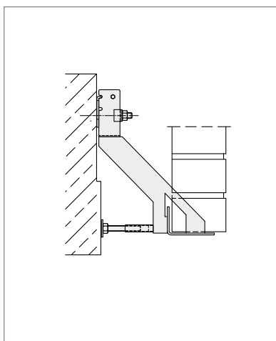
▲ Druckschraube \pm 15 mm justierbar
