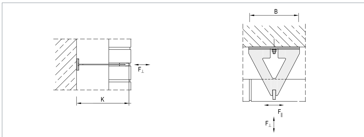
▲ MOSO® scaffold anchor GA-Q
