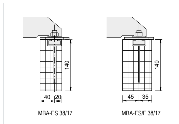
▲ MOSO® MBA-ES and MBA-ESF 38/17
