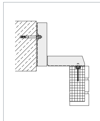
▲ FB-G, elevation below
