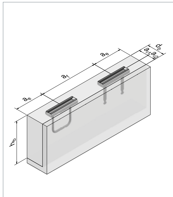
▲ Left MBA 38/18 ES, right MBA 38/17 ESF
